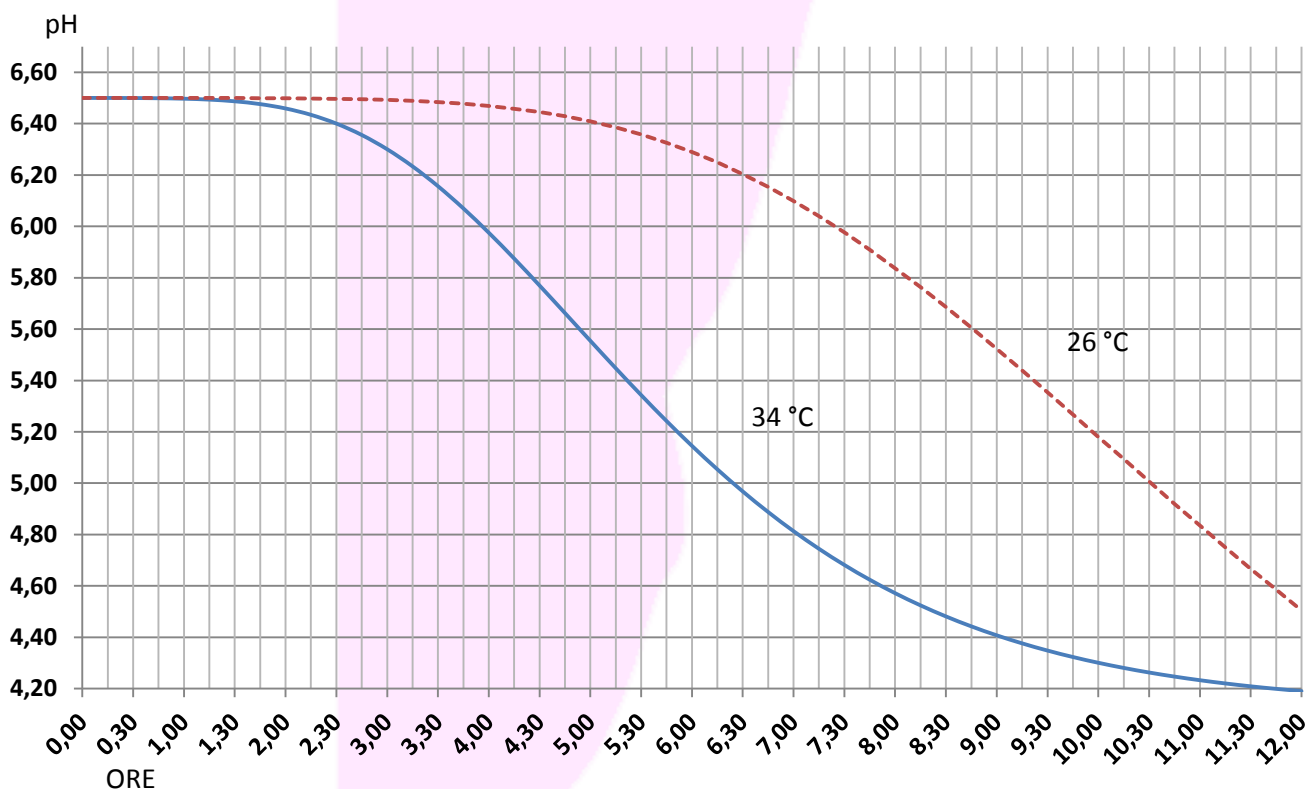
CURVA ACIDIFICAZIONE
